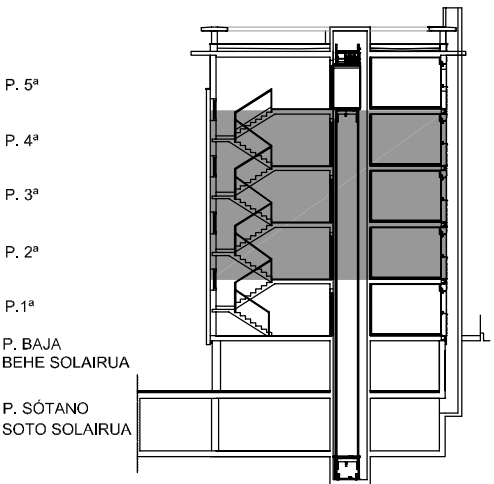
SUPERFICIES UTILES APROXIMADAS GUTXI GORA BEHERAKO AZALERA ERABILGARRIA
